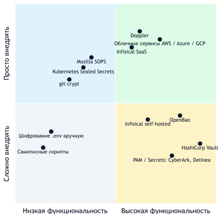
Рисунок 5 – Сравнение решений для управления секретами
